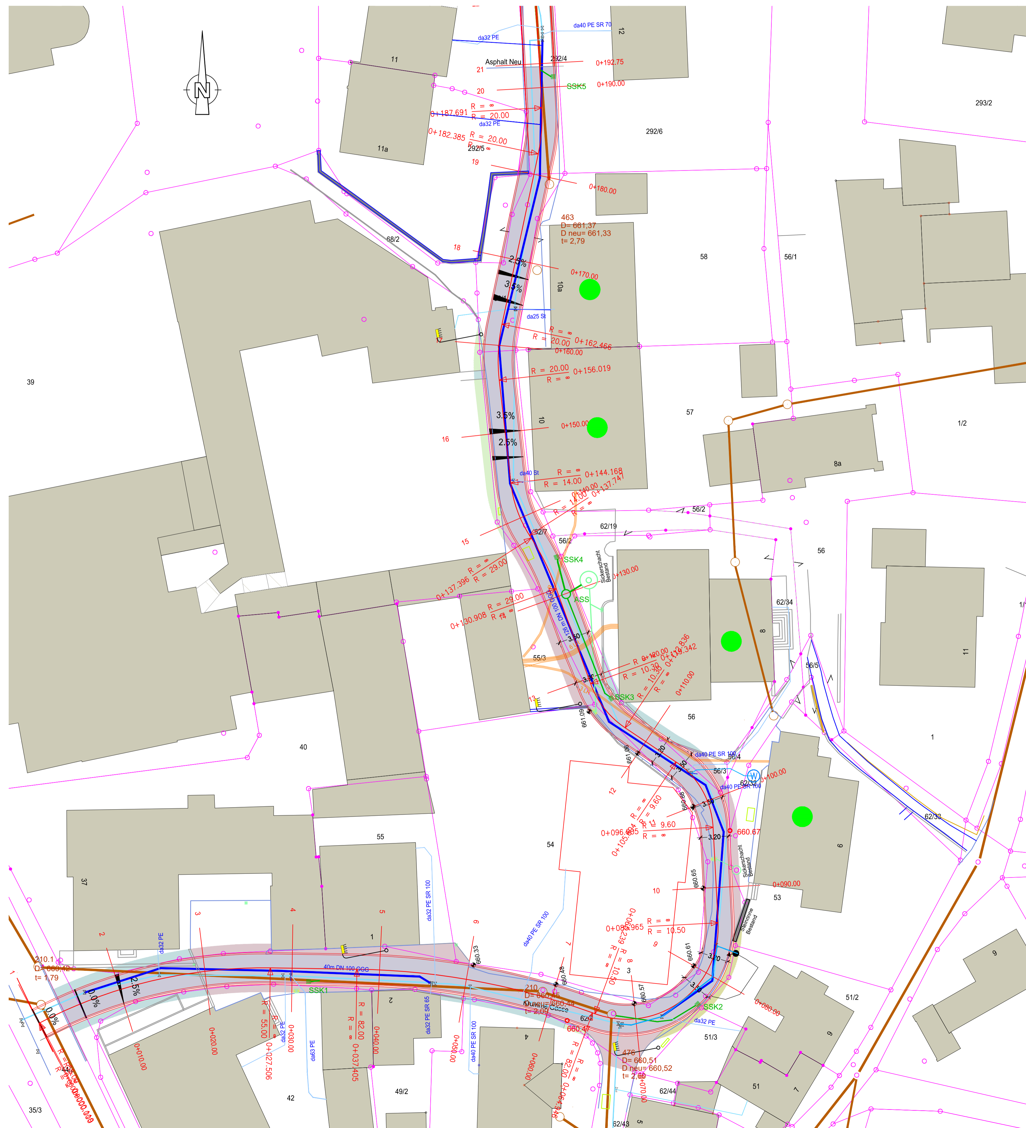
Lageplan M= 1 : 250
