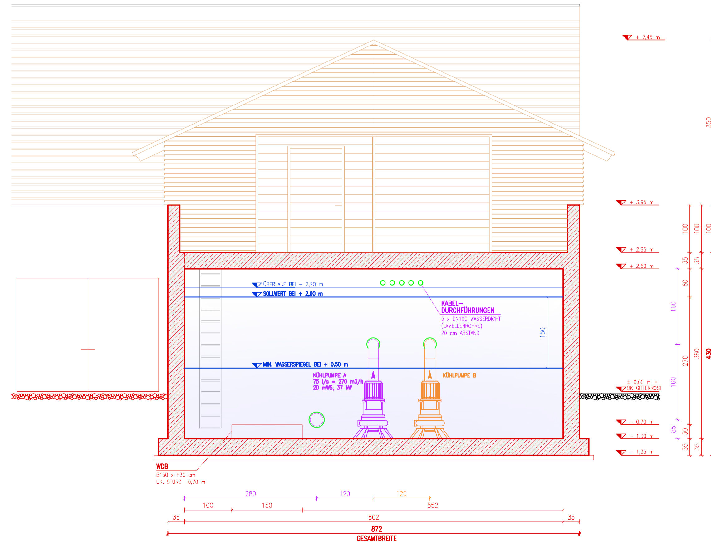
SCHNITT C-C M = 1 : 50
